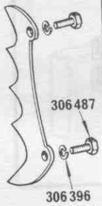
KIT - PART N° 474591
