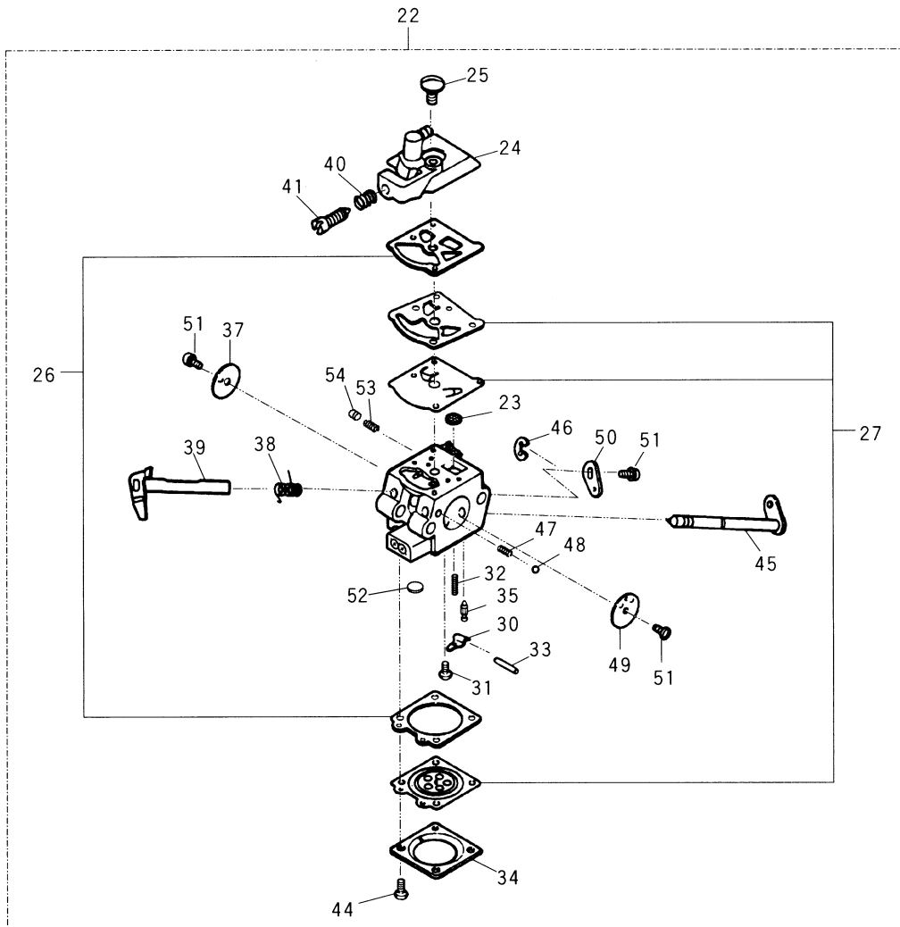
Fig.6 CARBURETOR
