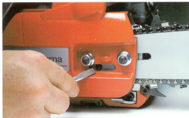
Kedjesträckare från sidan gör att det går snabbare och lättare att justera kedjespänningen.
