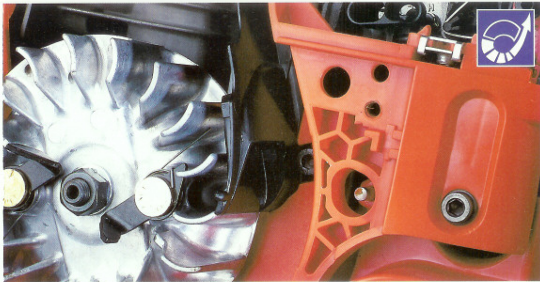
Air Injection renar effektivt insugningsluften, vilket ger jämnare gång, förlänger tiden mellan filterrengöringar och minskar slitaget på motorn.
